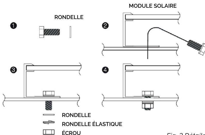
Fig. 3 Détails de montage
